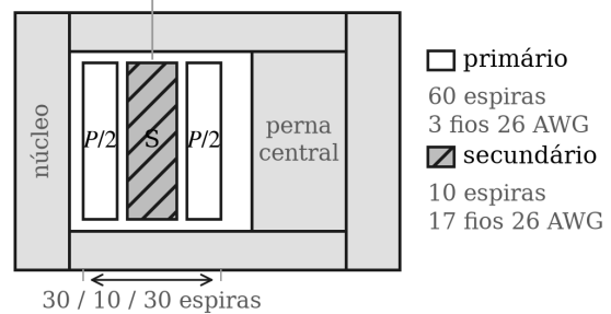
Fig. 14. Corte da janela do núcleo com a sequência de bobinagem intercalada, adotada para reduzir o efeito de proximidade e a indutância de dispersão.
