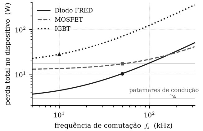
Fig. 7. Perda total nos três dispositivos comutados dos exemplos, em função da frequência. As linhas horizontais são os patamares de condução, independentes da frequência; a inclinação unitária em escala logarítmica é a assinatura da perda de comutação.
