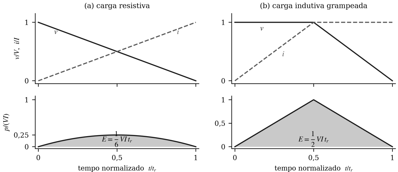
Fig. 1. Sobreposição de tensão e corrente durante a entrada em condução. Com carga resistiva as duas grandezas variam simultaneamente e a energia é um sexto do produto; com carga indutiva grampeada elas variam em sequência e a energia é a metade.
